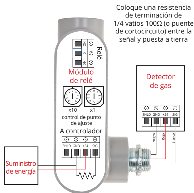
Figura 2 Configuración autónoma
