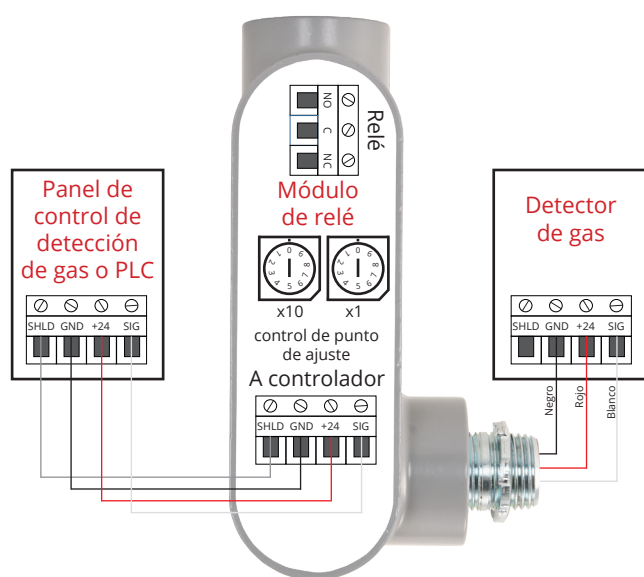
Figura 1 Configuración interconectada
